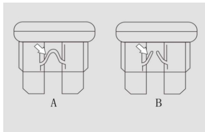
A: Нормальный предохранитель; B: Перегоревший предохранитель.
